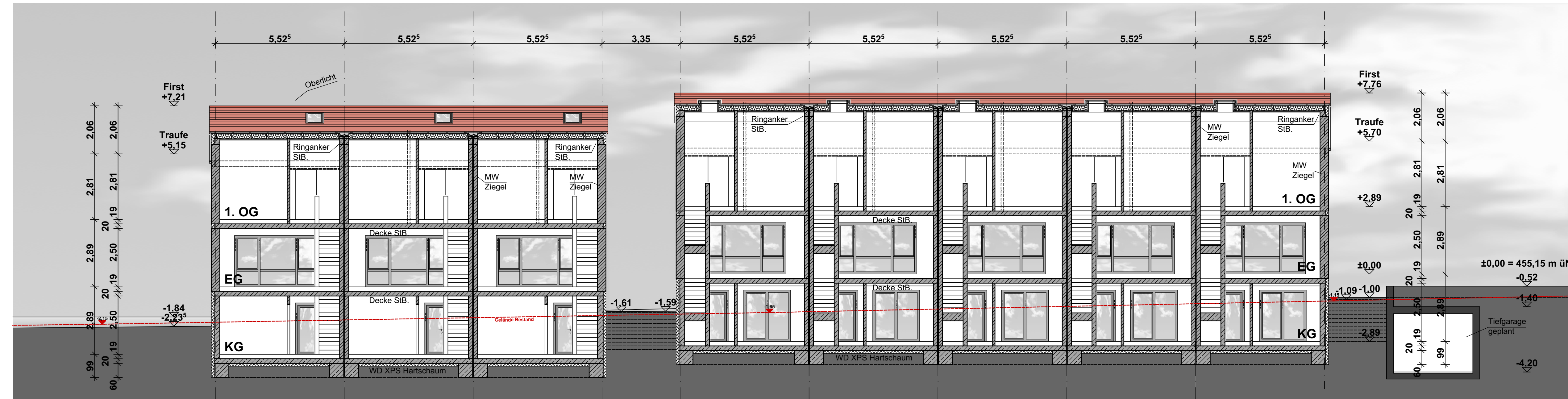
Schnitt 2
