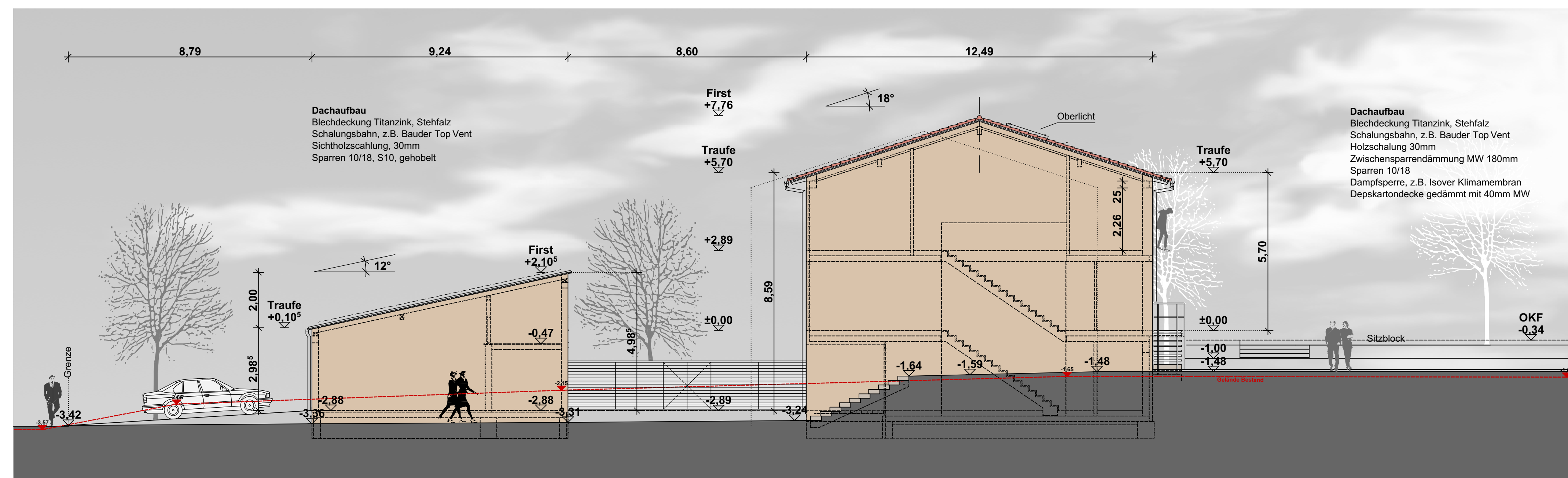
Ansicht Ost Garagen Baukörper 1
