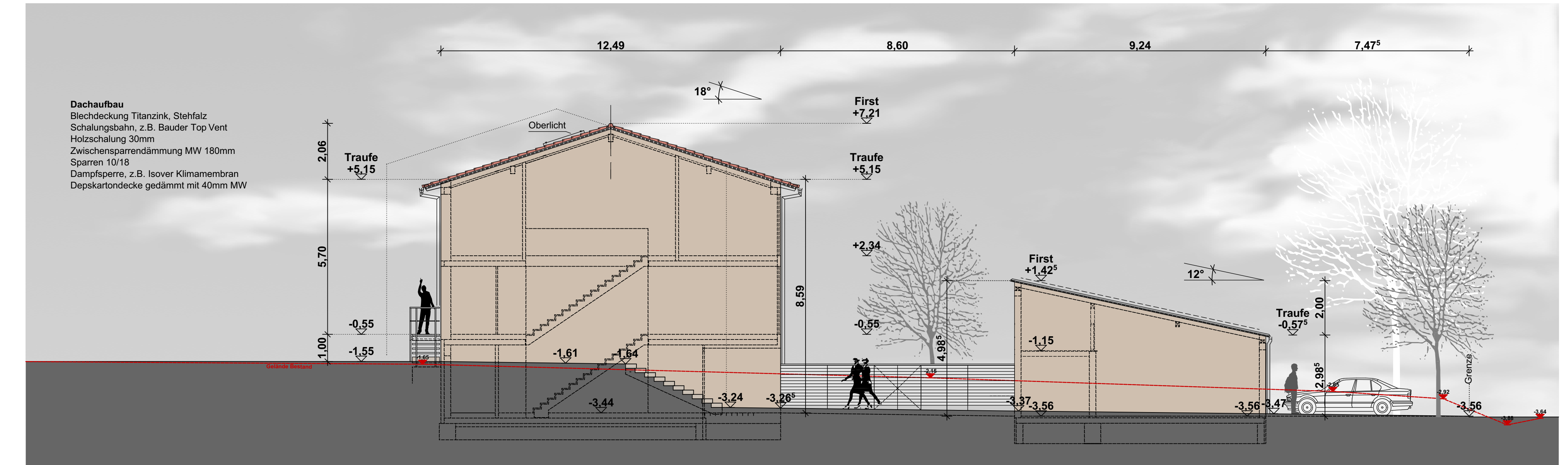
Ansicht West Baukörper 2
