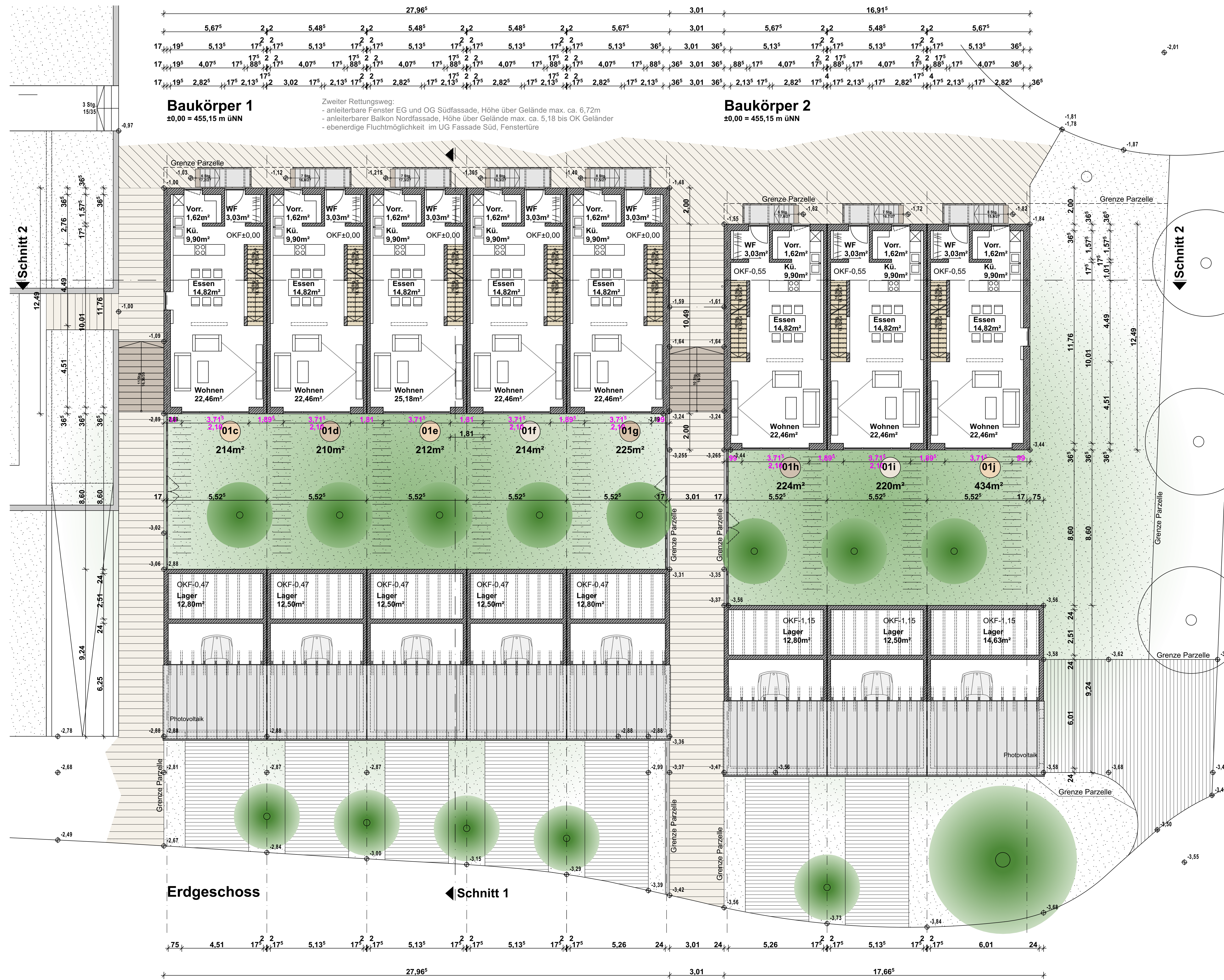
Erdgeschoss
