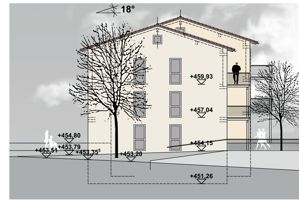
Ansicht Süd BK C
