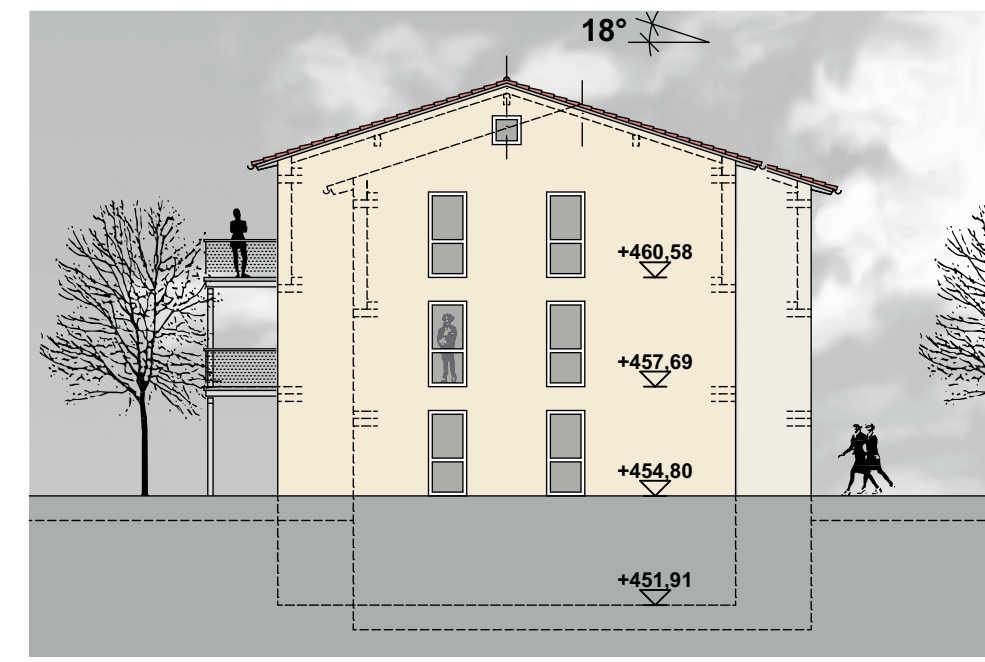
Ansicht Nord BK D
