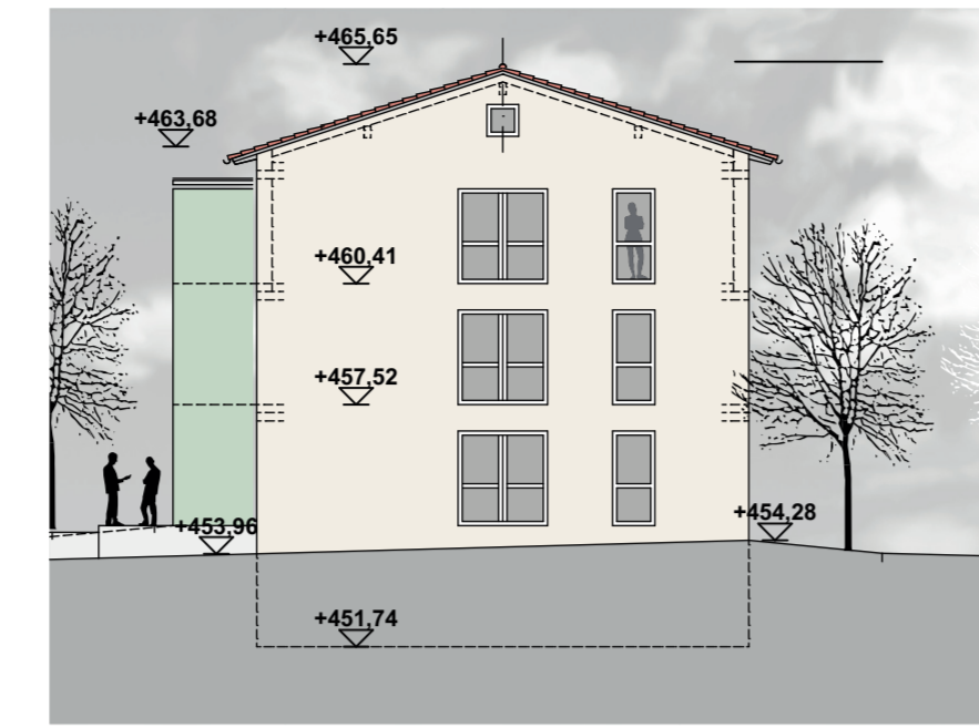
Ansicht West BK A
