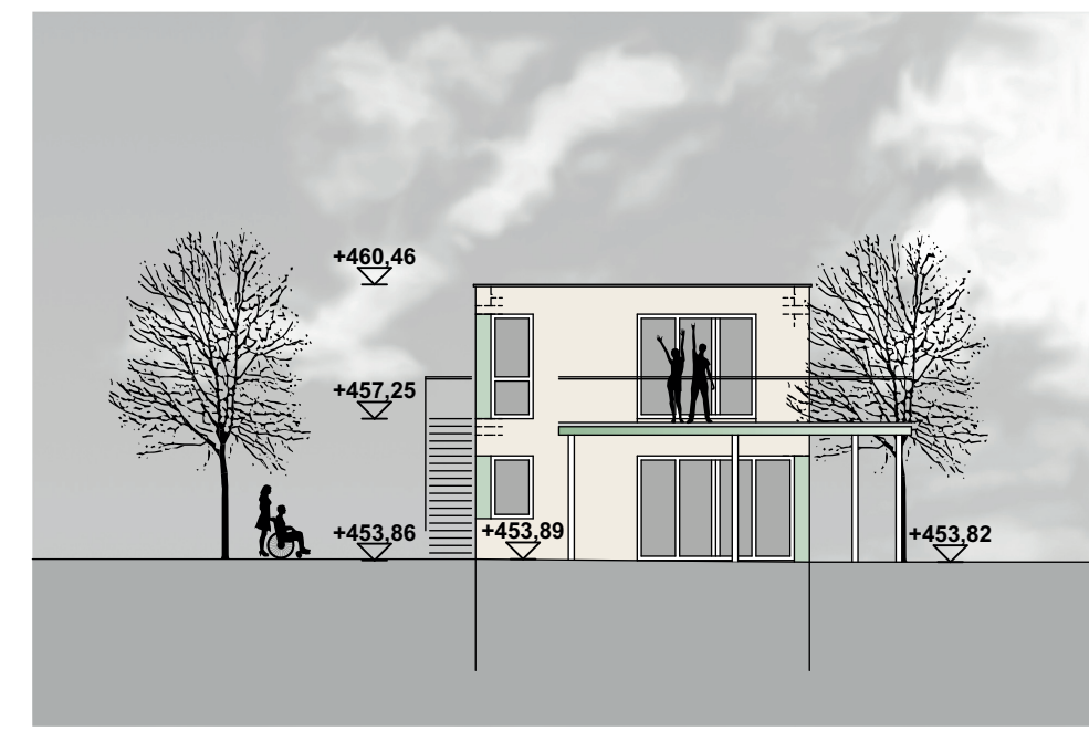
Ansicht West BK B
