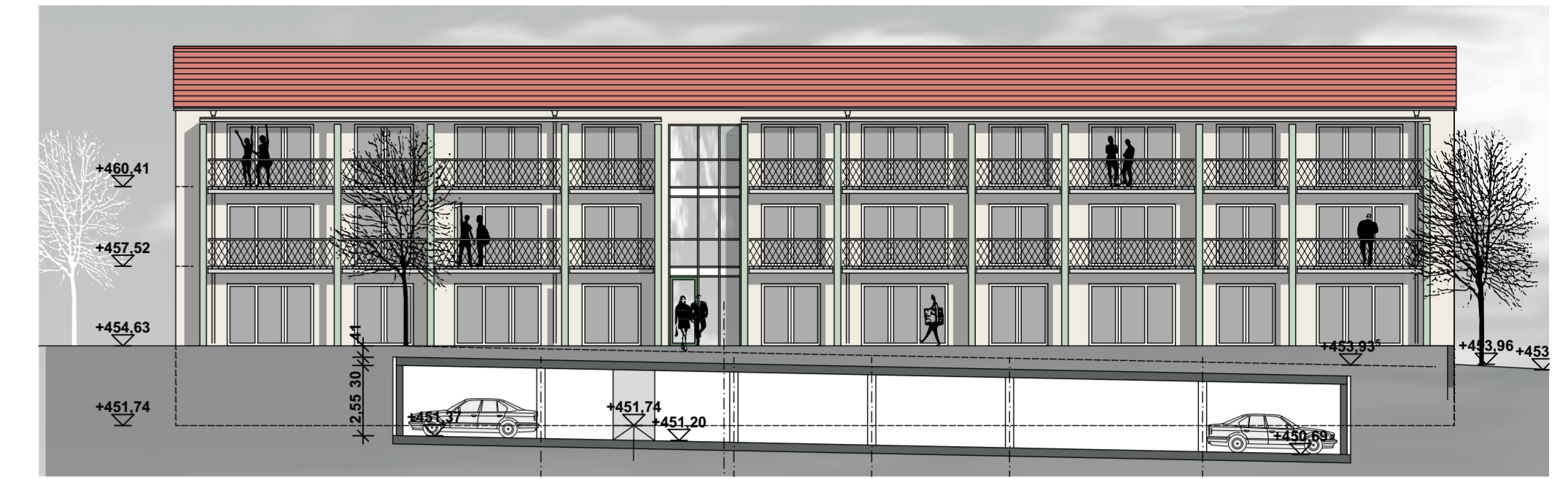
Ansicht Süd BK A
