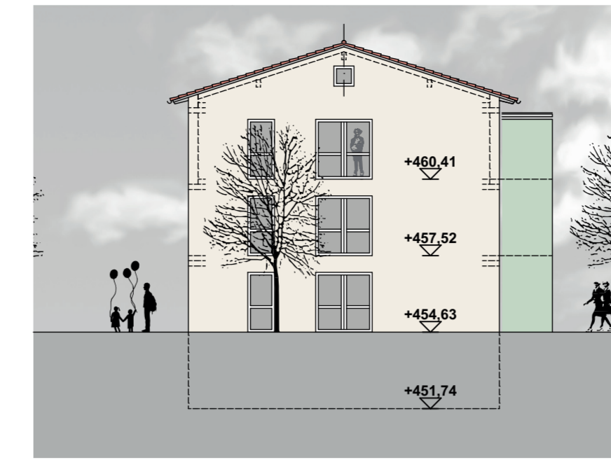
Ansicht Ost BK A
